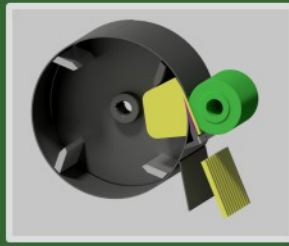
Schneiden von Streifen mit Trennmesser und oberen Kreismessern Cutting of strips with block knife and upper circular knives
