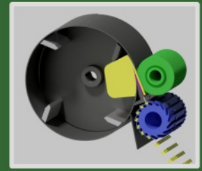
Schneiden von Würfeln mit Trennmesser, oberen Kreismessern und unteren Quermessern Cutting of cubes with block knife, upper circular knives and lower cross knives
